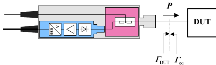
Bild 6-2 Korrektur der Wechselwirkungen zwischen Leistungsmesskopf und DUT
