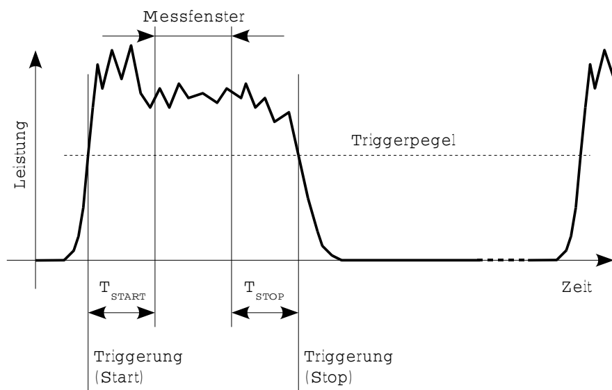
Bild 6-4 Wirkung von SENSe:TIMing:EXCLude:START und -:STOP im Burst Average -Modus
