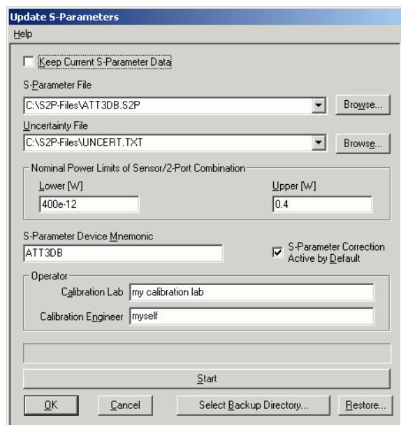
Bild 3-3 Dialogfenster für das Laden einer S-Parameter-Tabelle
