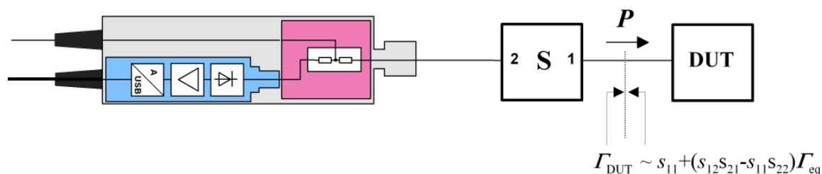
Bild 6-3 Korrektur der Wechselwirkungen zwischen Leistungsmesskopf, DUT und S-Parameter-Device
