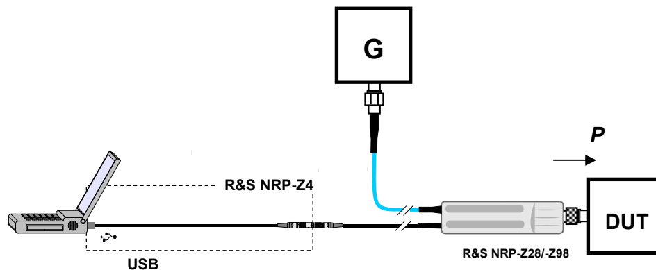
Bild 1-3 Leistungsmessung am PC mit dem passiven USB-Adapter R&S NRP-Z4
