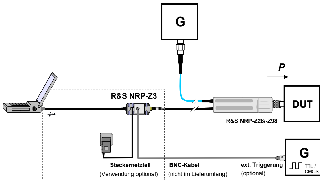
Bild 1-4 Leistungsmessung am PC mit dem aktiven USB-Adapter R&S NRP-Z3
